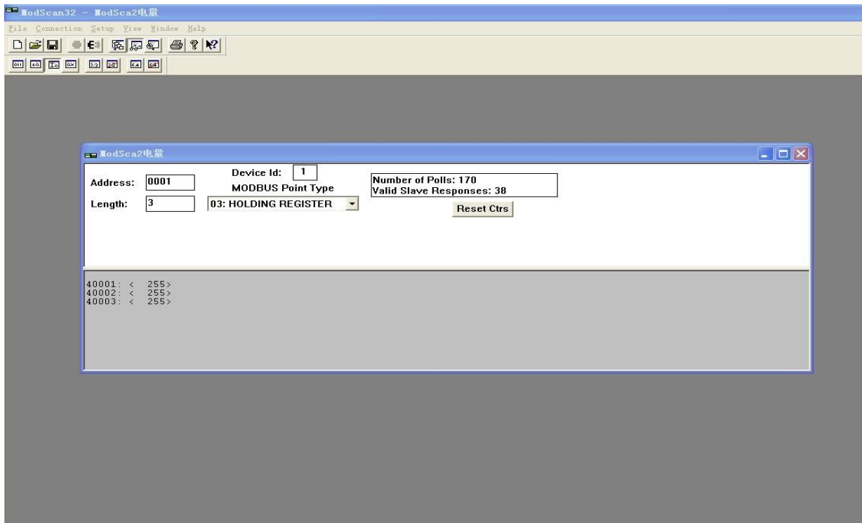
(1) 03 代码测试图
