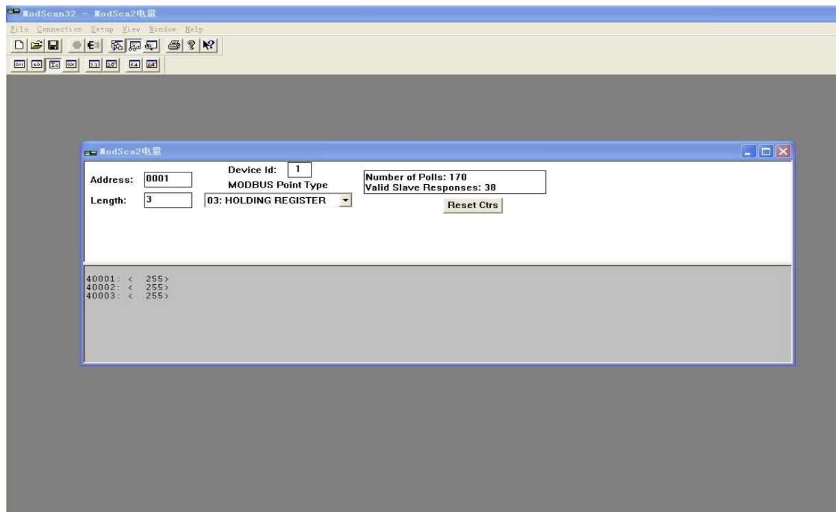
(1) 03 代码测试图
