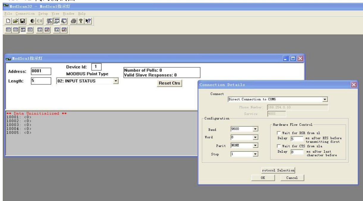
(1) 02 代码测试图
